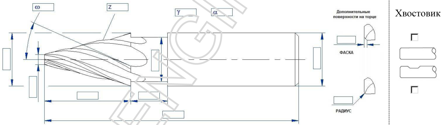
ω - угол подъема режущей кромки; z - число зубьев; γ - передний угол; α - задний угол
